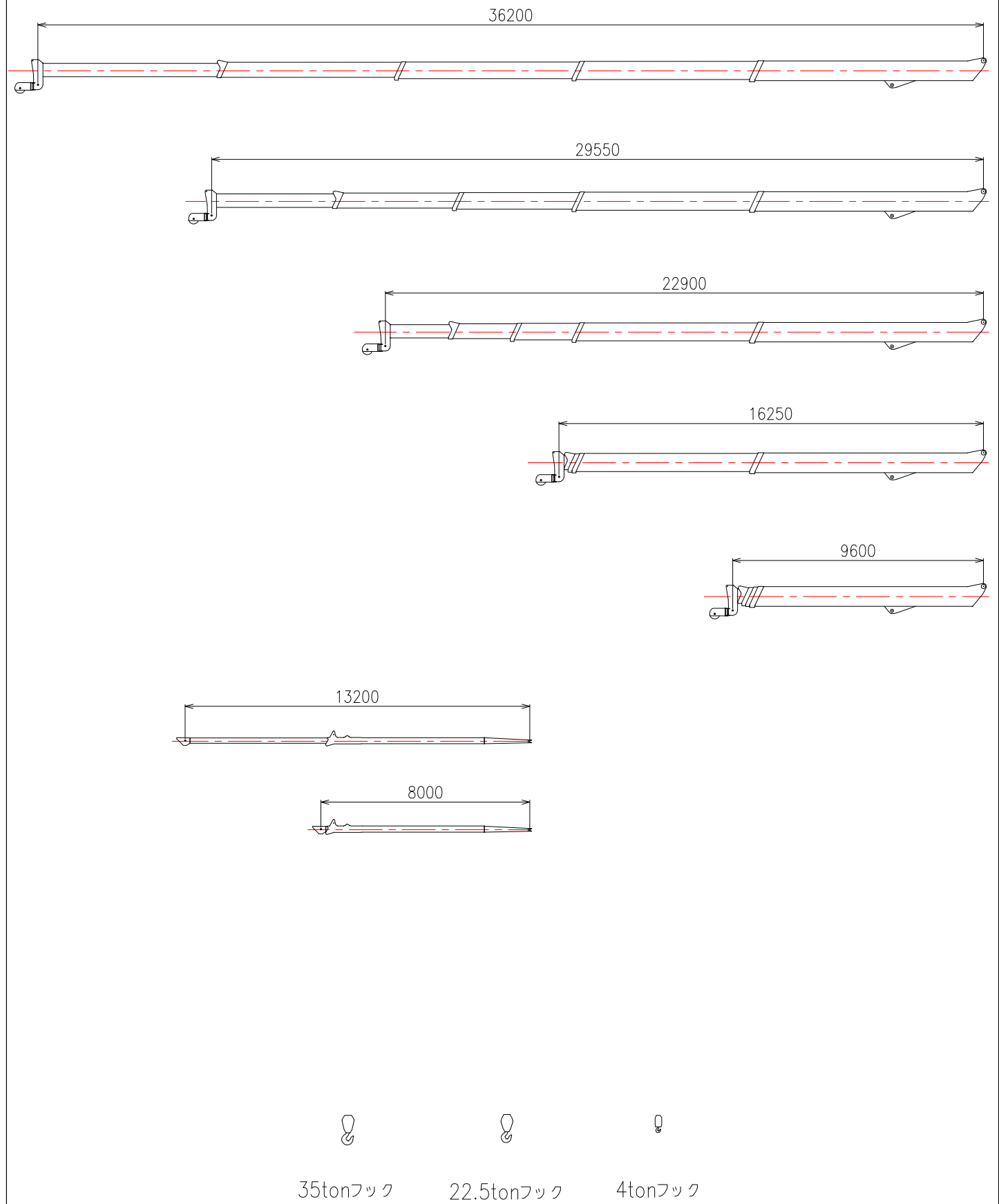
参考図 (ブーム・フック) ブロック
